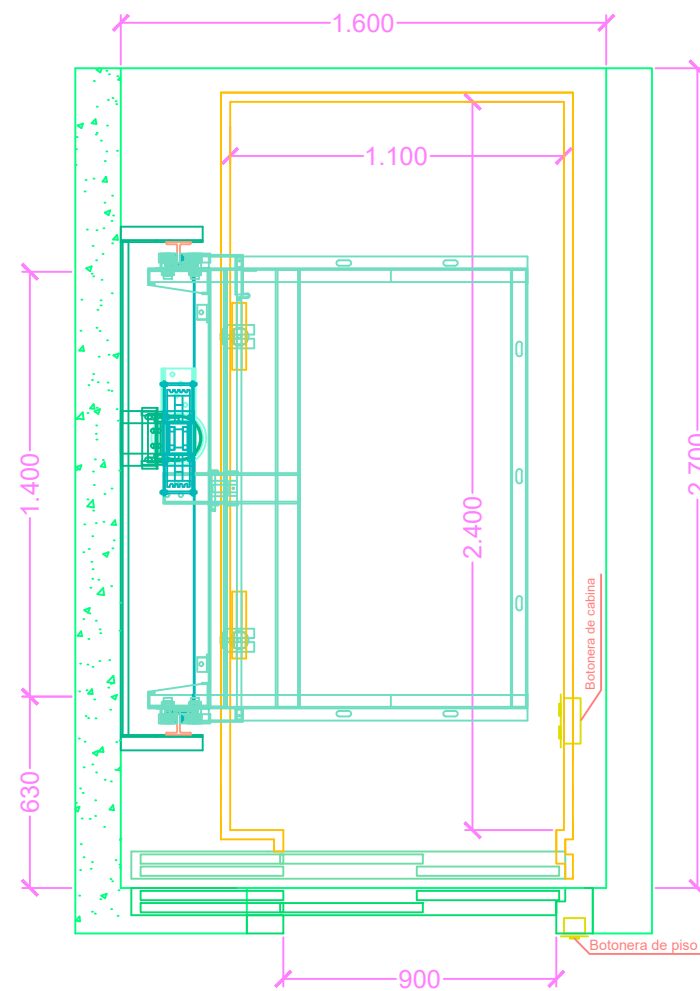
ENTRADAS VISTA EN PLANTA PASADIZO
