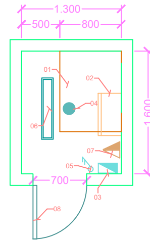
VISTA EN PLANTA SALA DE MAQUINA
